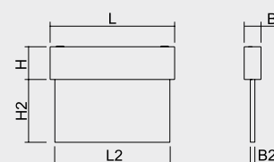
Universalmontage (Deckenaufbau)
